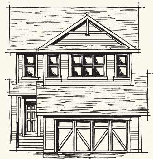
Elevation A
